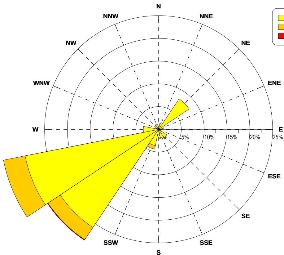
KIERUNKOWO-PRĘDKOŚCIOWA RÓŻA WIATRÓW BORUCINO
