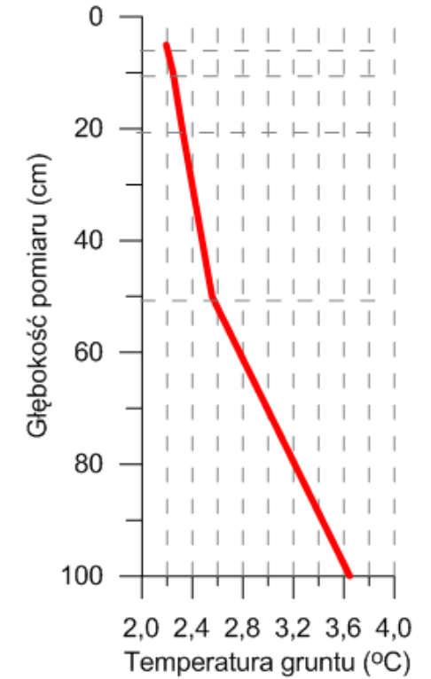
Średnia miesięczna temperatura gruntu Borucino - luty 2019
