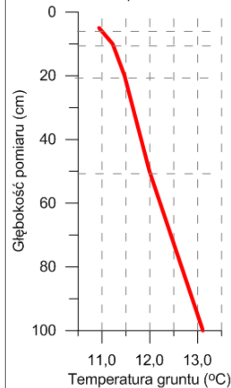
Średnia miesięczna temperatura gruntu Borucino - październik 2018
