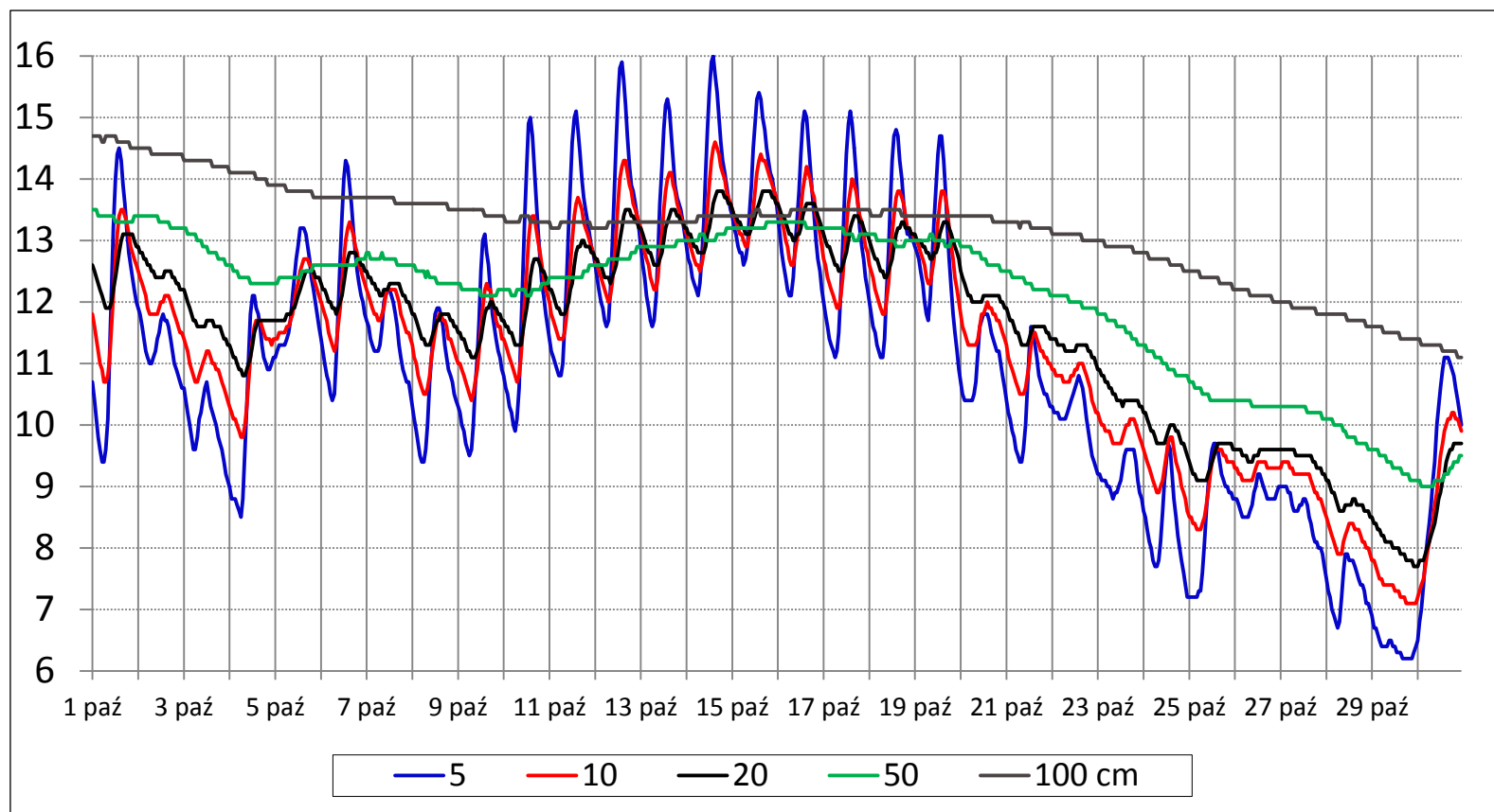
Średnia miesięczna temperatura gruntu Borucino - październik 2018
