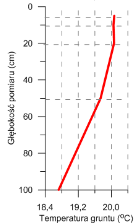
Średnia miesięczna temperatura gruntu Borucino - sierpień 2018
