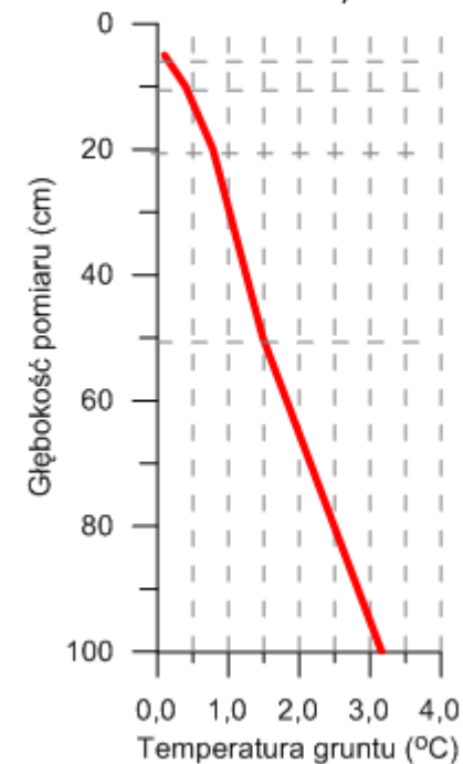
Średnia miesięczna temperatura gruntu Borucino - luty 2018
