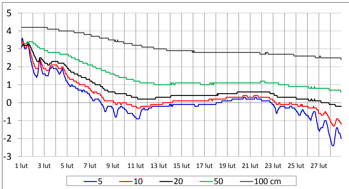
Średnia miesięczna temperatura gruntu Borucino - luty 2018
