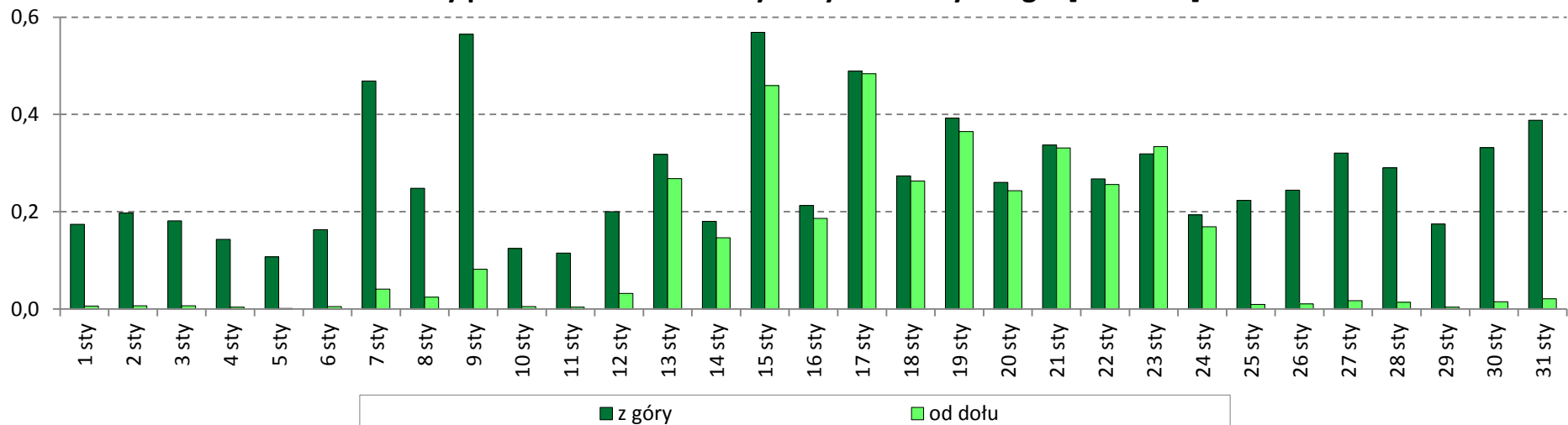
Sumy promieniowania fotosyntetycznie aktywnego [ \text{mol} \cdot \text{m}^{-2} ]
