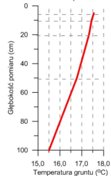
Średnia miesięczna temperatura gruntu Borucino - lipiec 2017
