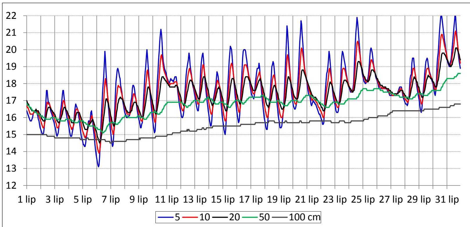
Średnia miesięczna temperatura gruntu Borucino - lipiec 2017
