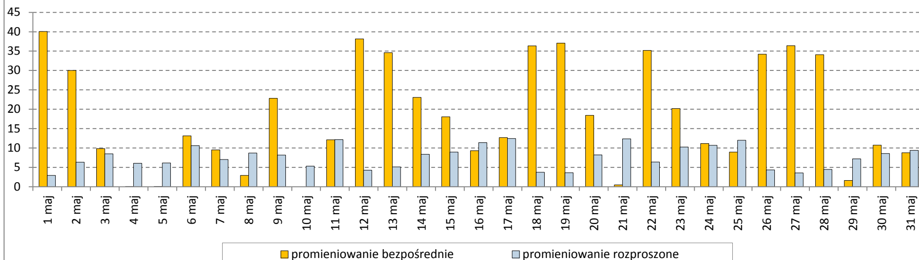
Sumy dobowe energii promieniowania bezpośredniego i rozproszonego [ \text{MJ} \cdot \text{m}^{-2} ]
