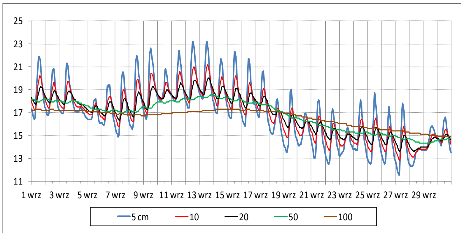
Średnia miesięczna temperatura gruntu (°C) - wrzesień 2016
