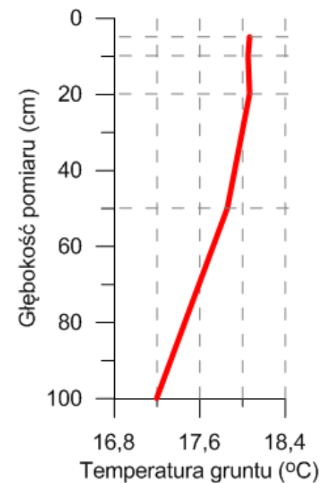
Średnia miesięczna temperatura gruntu (°C) - wrzesień 2016
