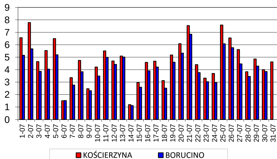
TEMPERATURA PRZY GRUNCIE - ODCHYLENIE STANDARDOWE
