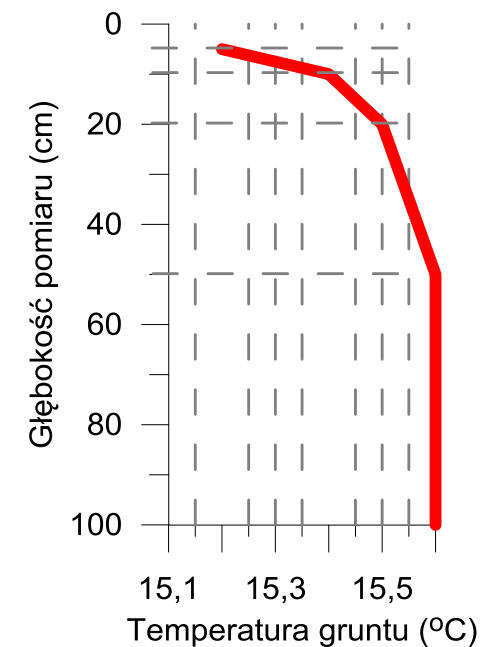
Średnia miesięczna temperatura gruntu - wrzesień 2015
