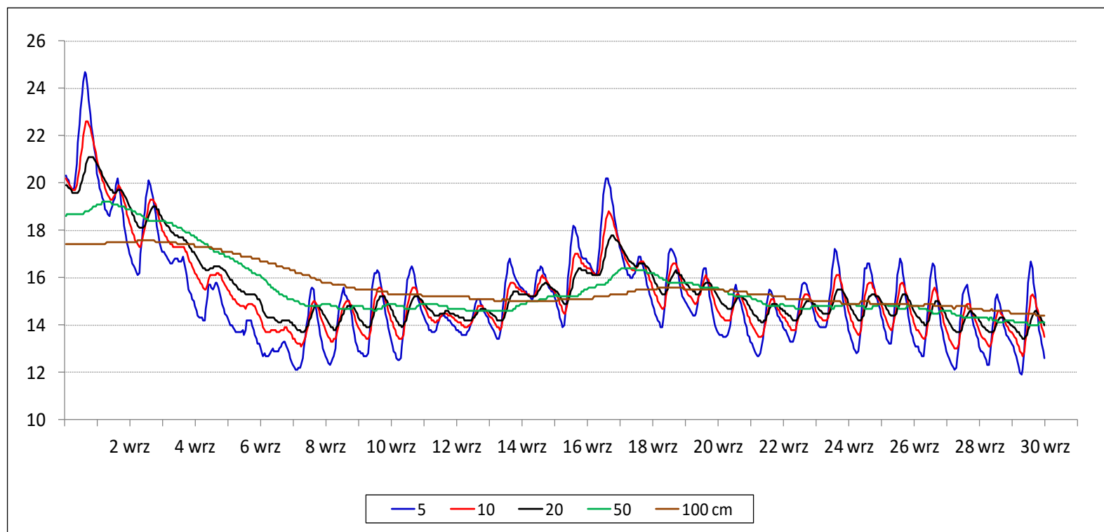
Średnia miesięczna temperatura gruntu - wrzesień 2015
