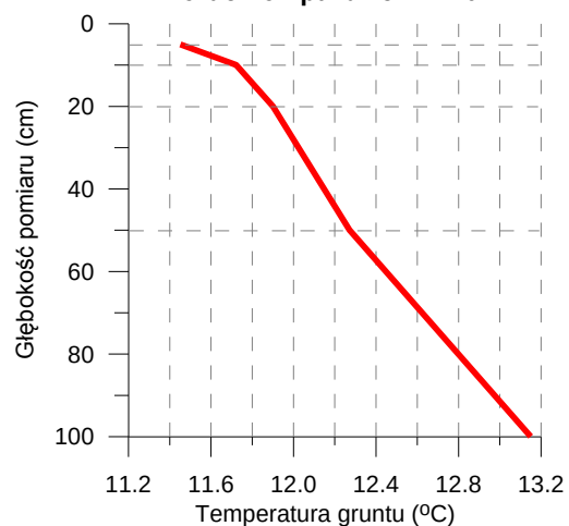
Średnia miesięczna temperatura gruntu Borucino - październik 2014
