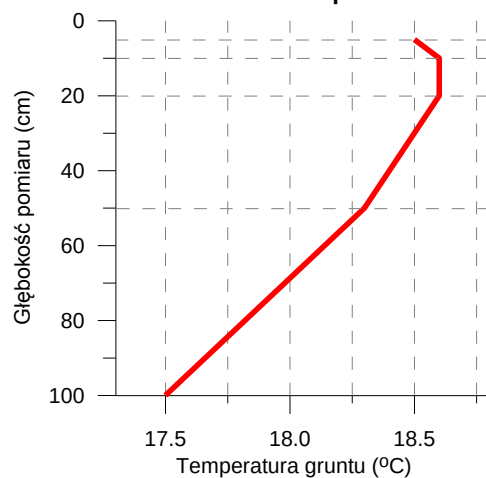
Średnia miesięczna temperatura gruntu Borucino - sierpień 2014
