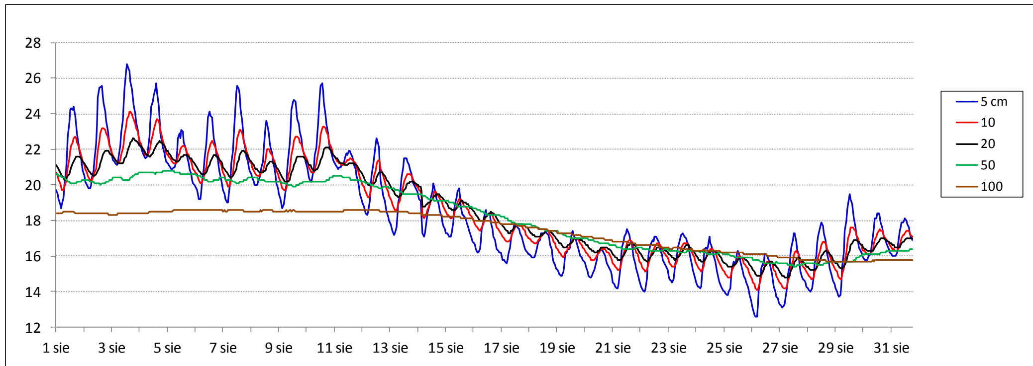
Średnia miesięczna temperatura gruntu Borucino - sierpień 2014
