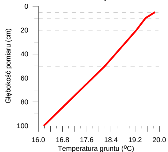
Średnia miesięczna temperatura gruntu Borucino - lipiec 2014
