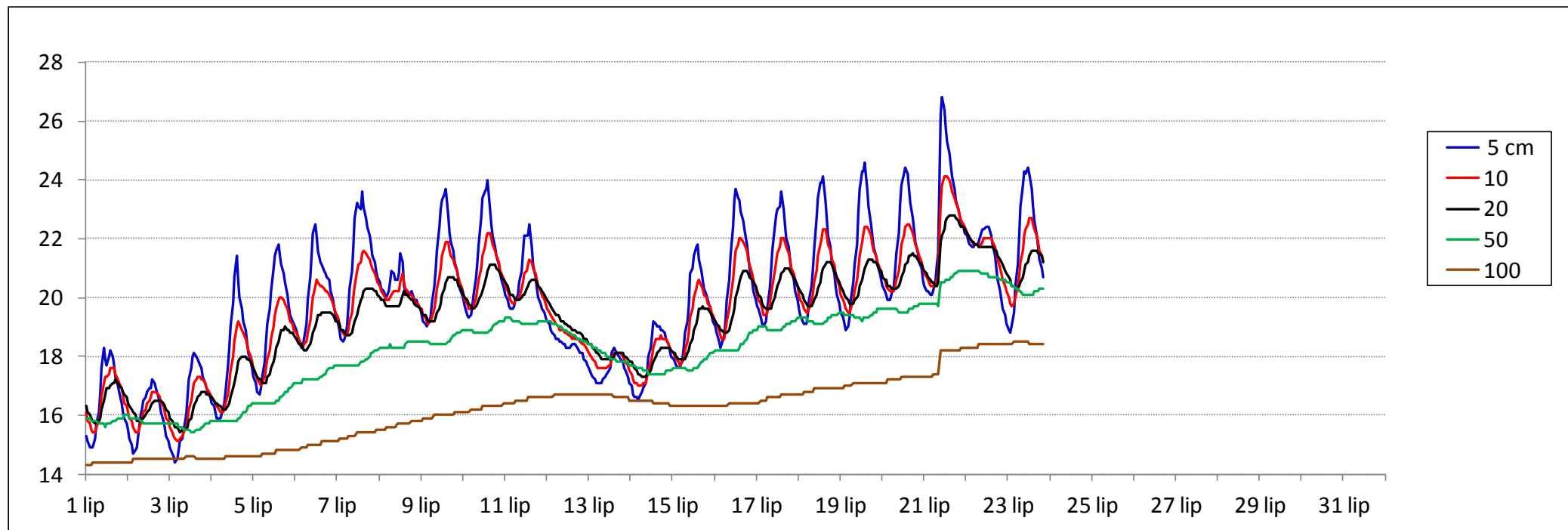
Średnia miesięczna temperatura gruntu Borucino - lipiec 2014
