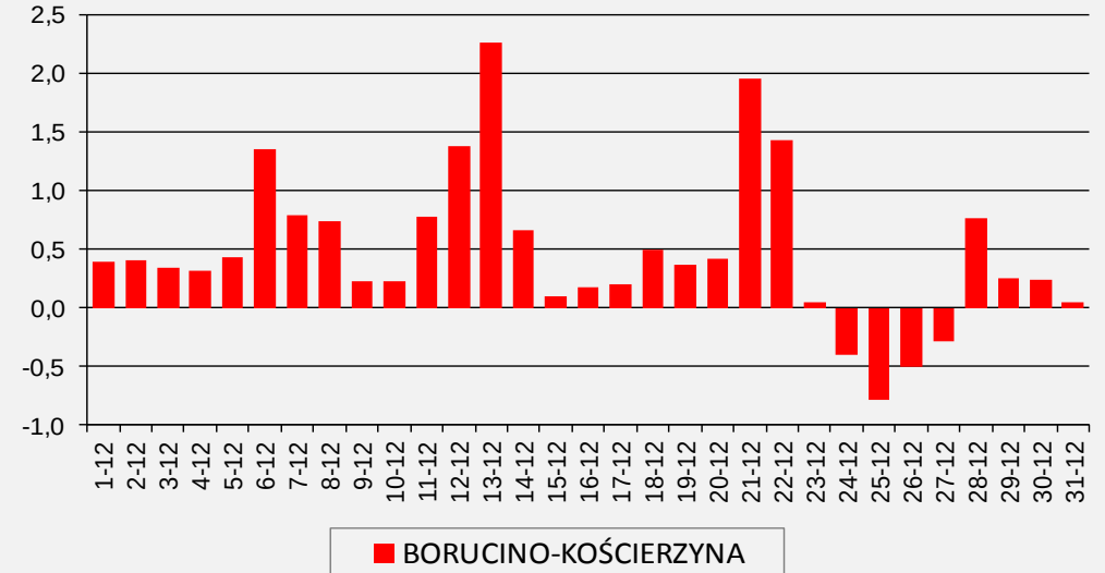
TEMPERATURA POWIETRZA PRZY GRUNCIE - RÓŻNICE
