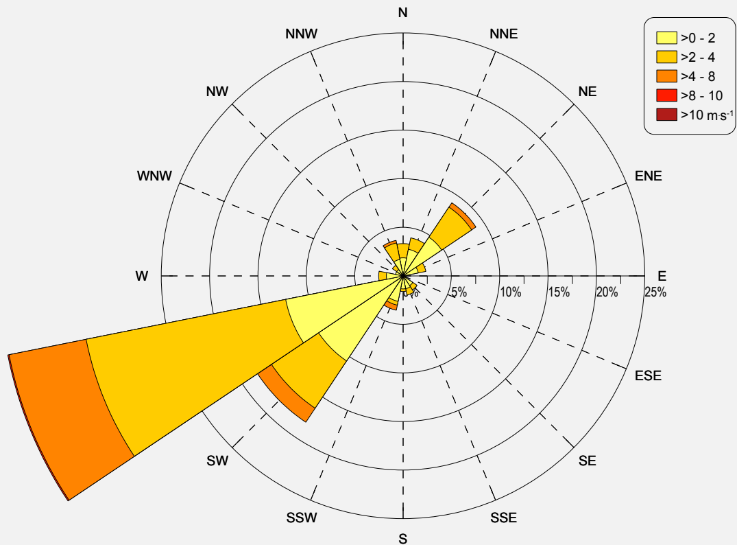
KIERUNKOWO-PRĘDKOŚCIOWA RÓŻA WIATRÓW BORUCINO
