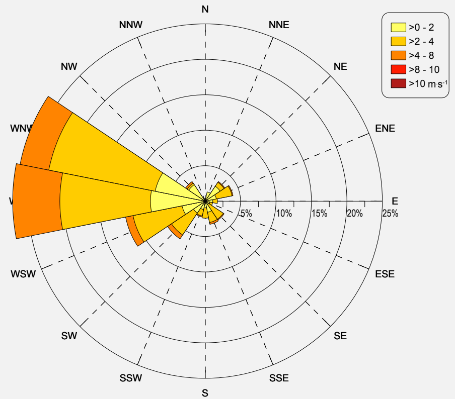
KIERUNKOWO-PRĘDKOŚCIOWA RÓŻA WIATRÓW KOŚCIERZYNA
