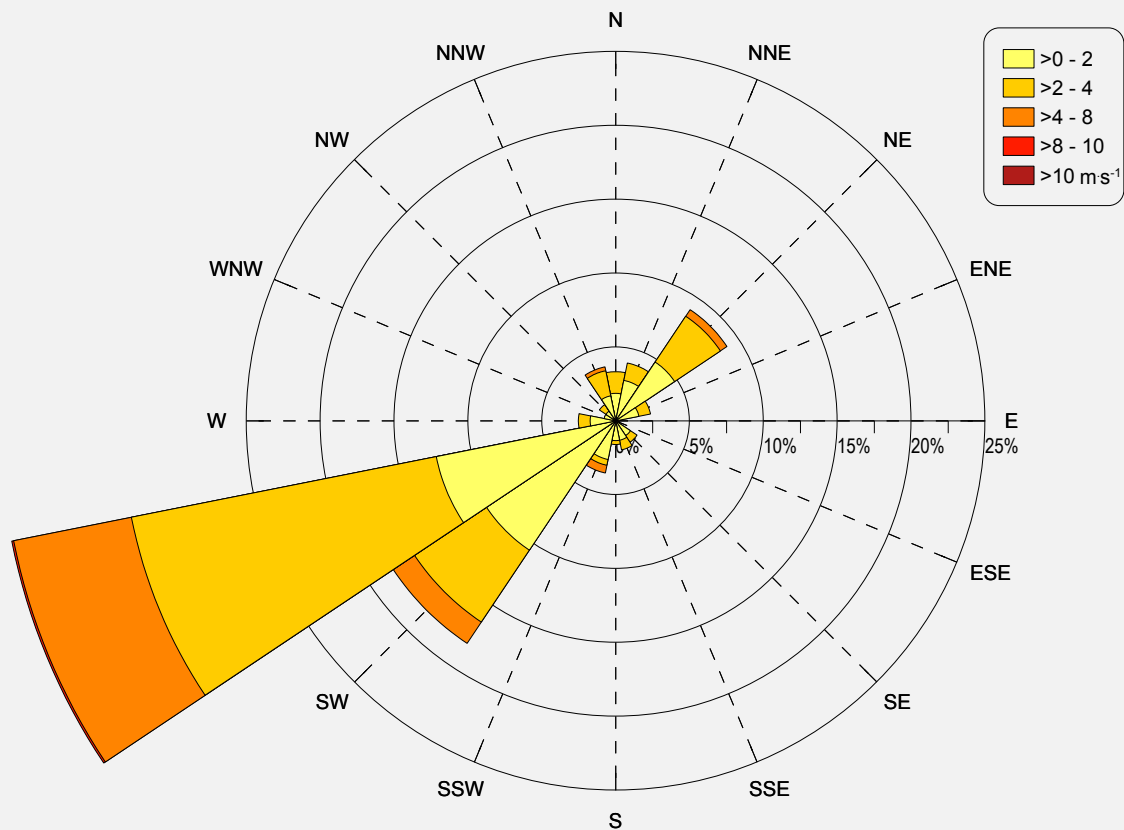
KIERUNKOWO-PRĘDKOŚCIOWA RÓŻA WIATRÓW BORUCINO
