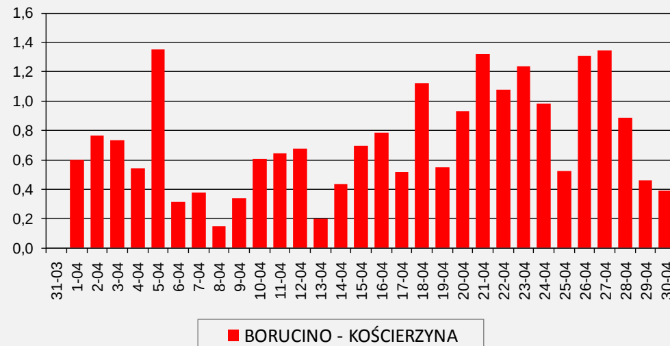
TEMPERATURA POW. - ODCHYLENIE STANDARDOWE RÓŻNIC
