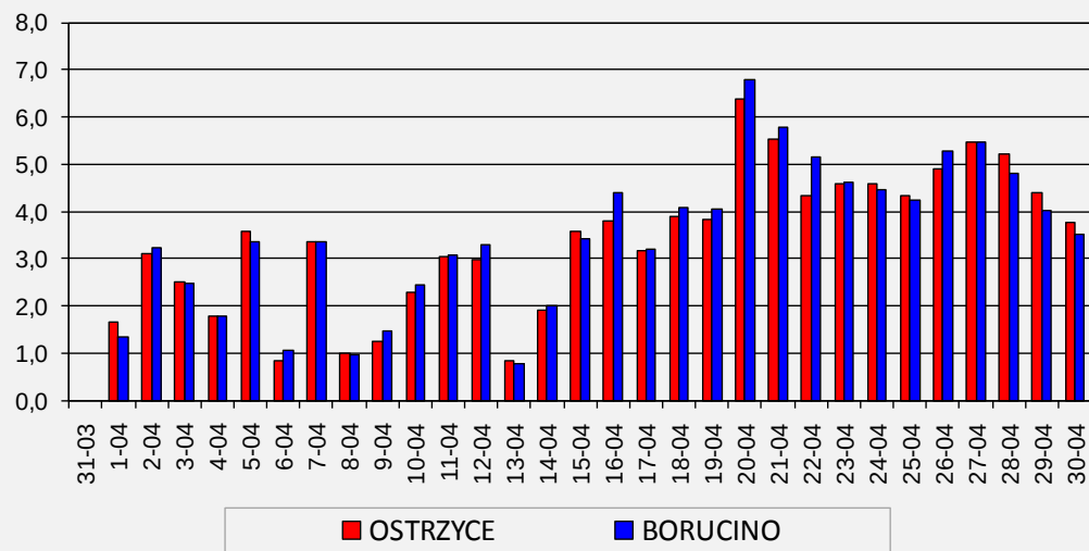
TEMPERATURA POWIETRZA - ODCHYLENIE STANDARDOWE
