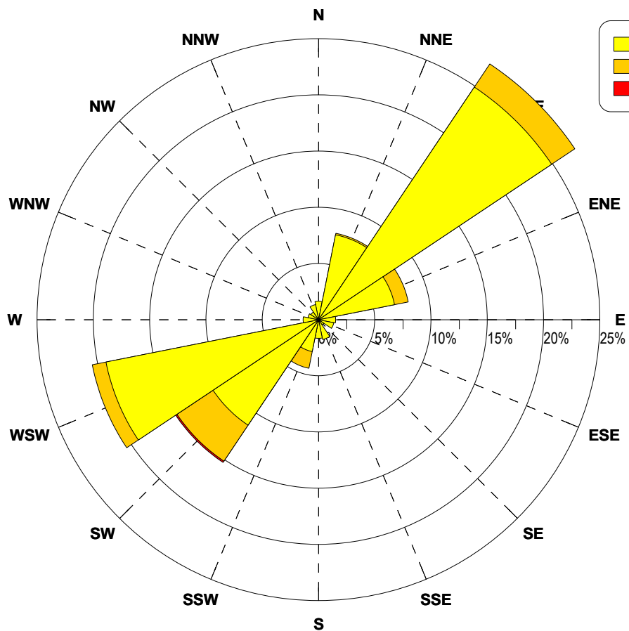
KIERUNKOWO-PRĘDKOŚCIOWA RÓŻA WIATRÓW BORUCINO
